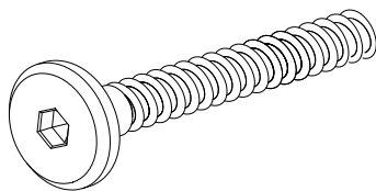
3x M6x40mm
